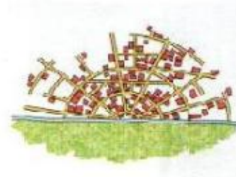
CITTA' VENTAGLIO
