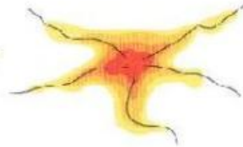
CITTA' STELLARE
